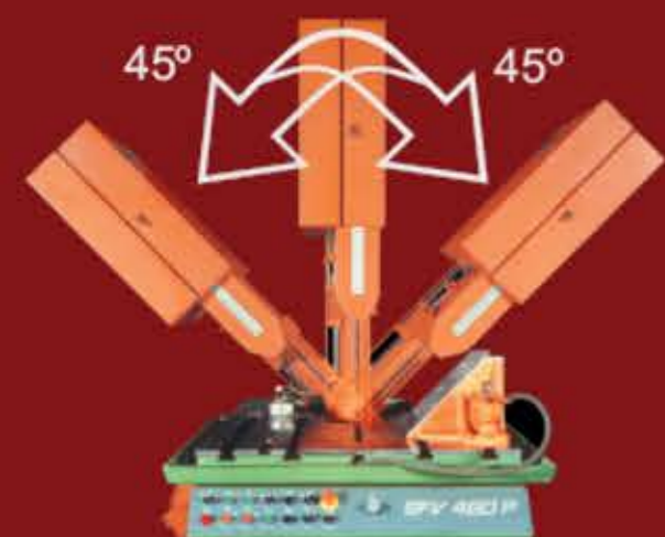
Ajuste hidráulico do ângulo de corte Leitura digital com encoder *Opcional
